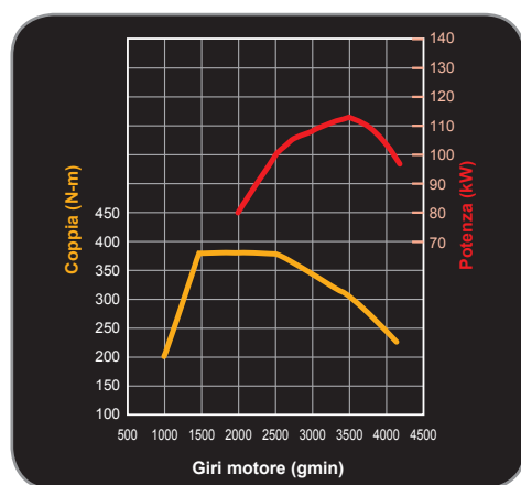
2.4-litri Turbodiesel DOHC DI-D (113 KW/3.500 gmin, 380 N-m/1.500-2.500 gmin)
